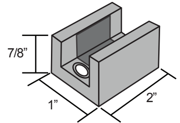
Door Guide
