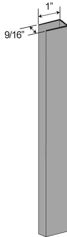
Hinge Jamb
